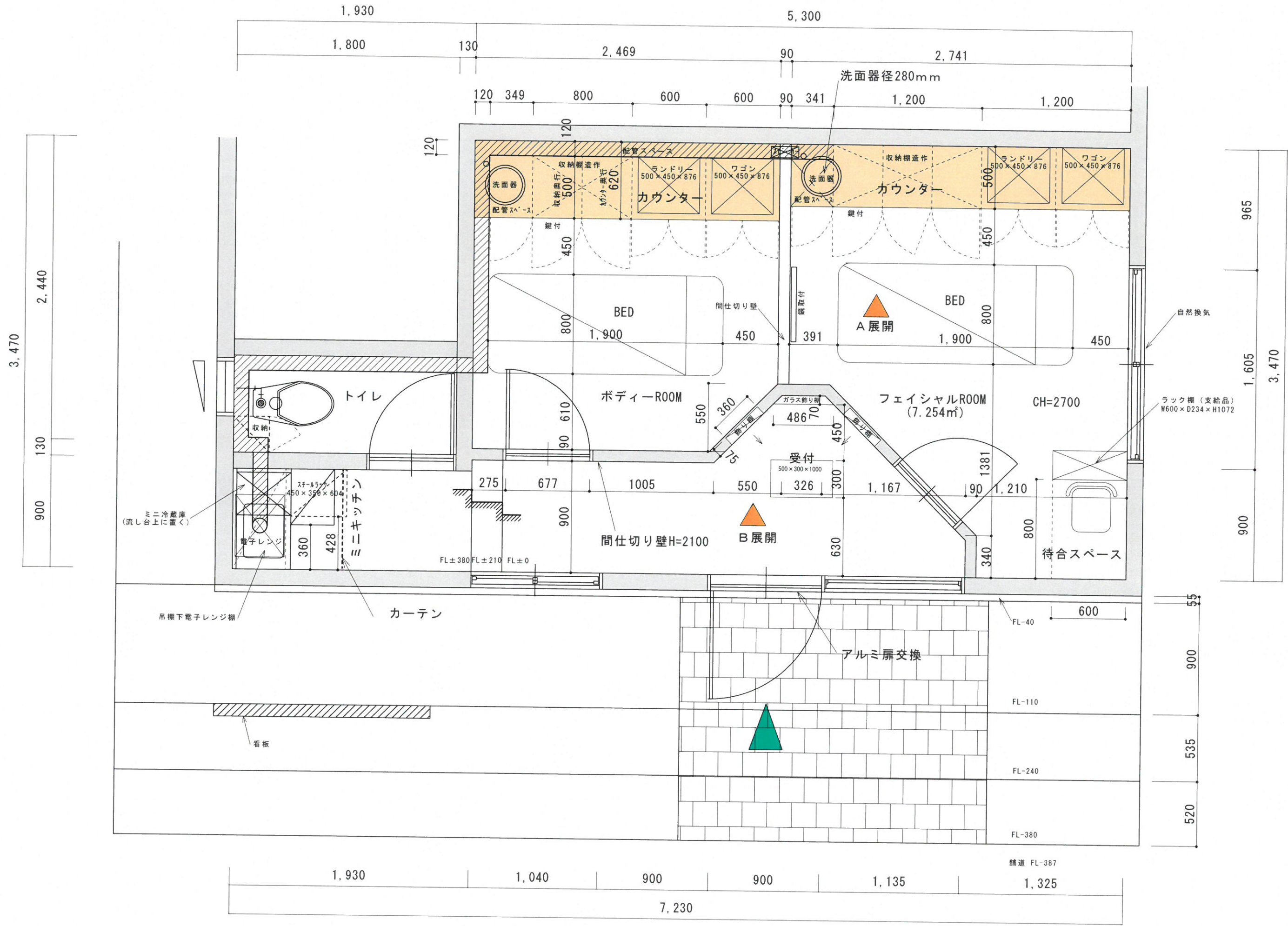
平面図 S=1/30
