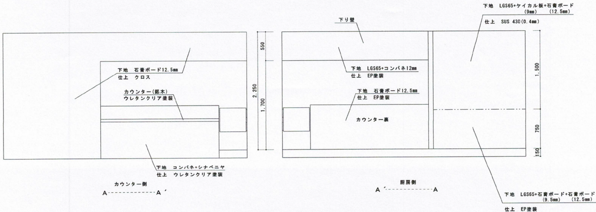
厨房 間仕切壁/下り壁/袖壁 立面図
