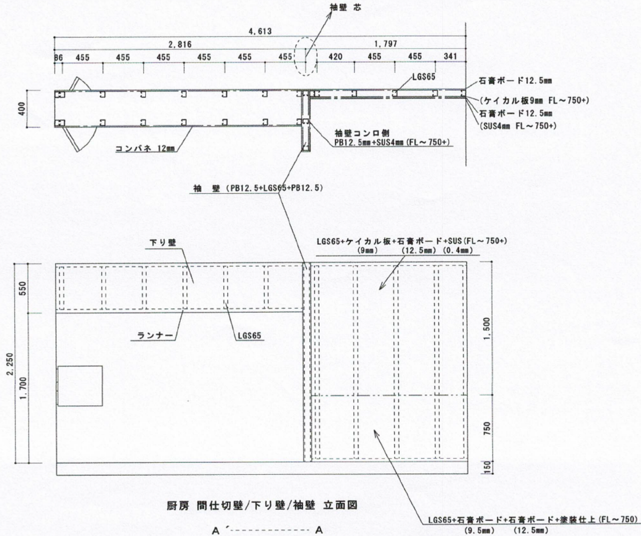
厨房 間仕切壁/下り壁/袖壁 上面図
