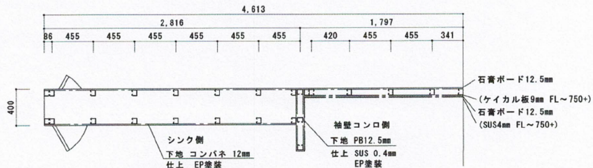
厨房 間仕切壁/下り壁/袖壁 上面図
