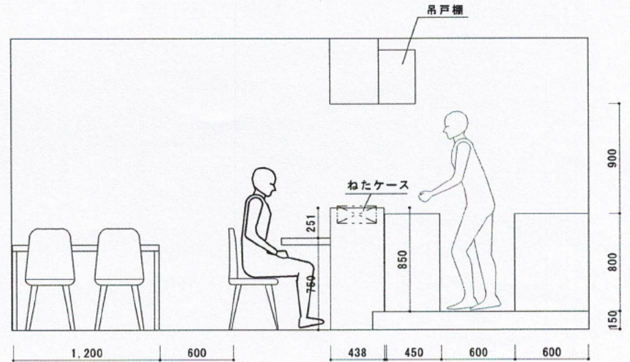
カウンター/厨房 断面
