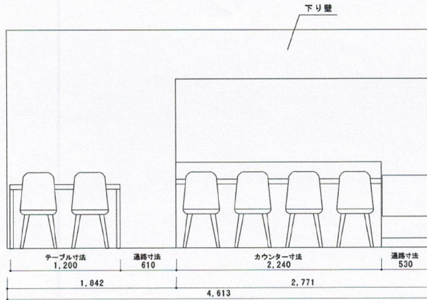
カウンター正面
