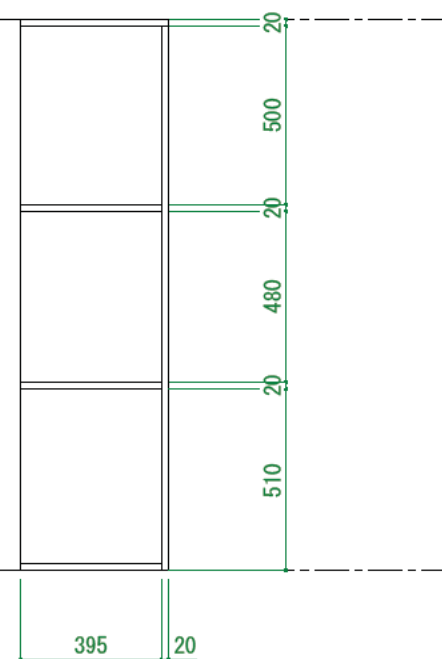
A 断面図
