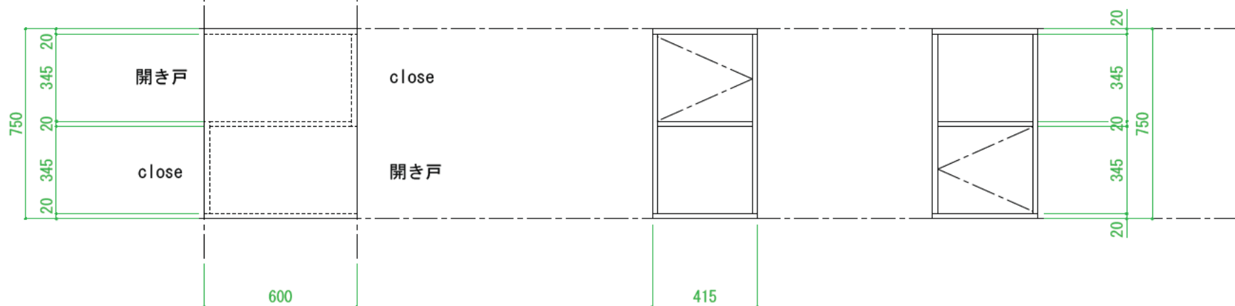
A-断面図
