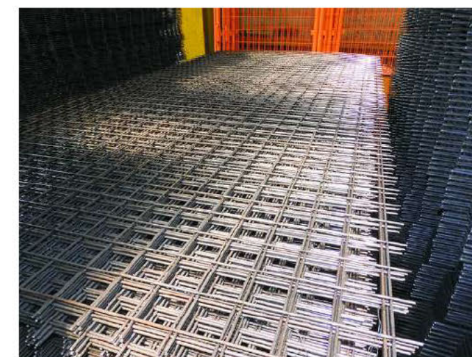
ワイヤメッシュ+錆止め塗装 (グレー色)
