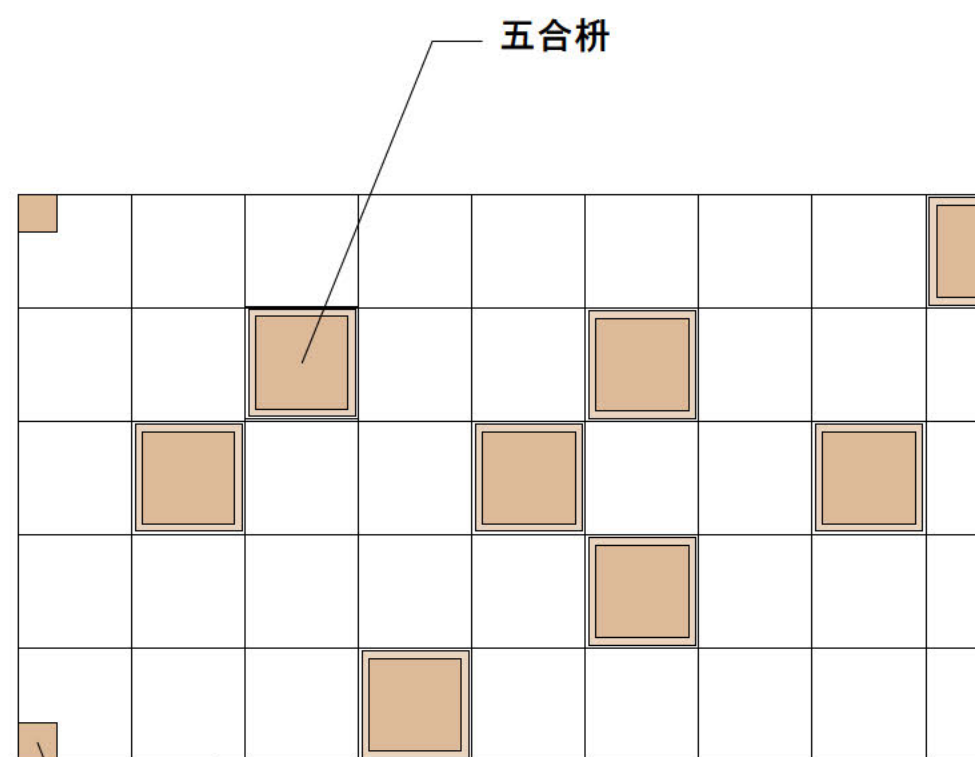
五合枧 ワイヤメッシュ+錆止め塗装 (グレー色) ワイヤ固定部材 (木製)
