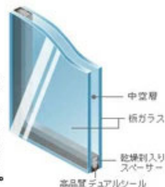
複層ガラス構造図
