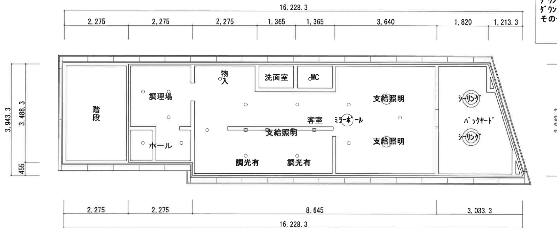
3階 天井伏図 S:1/70
