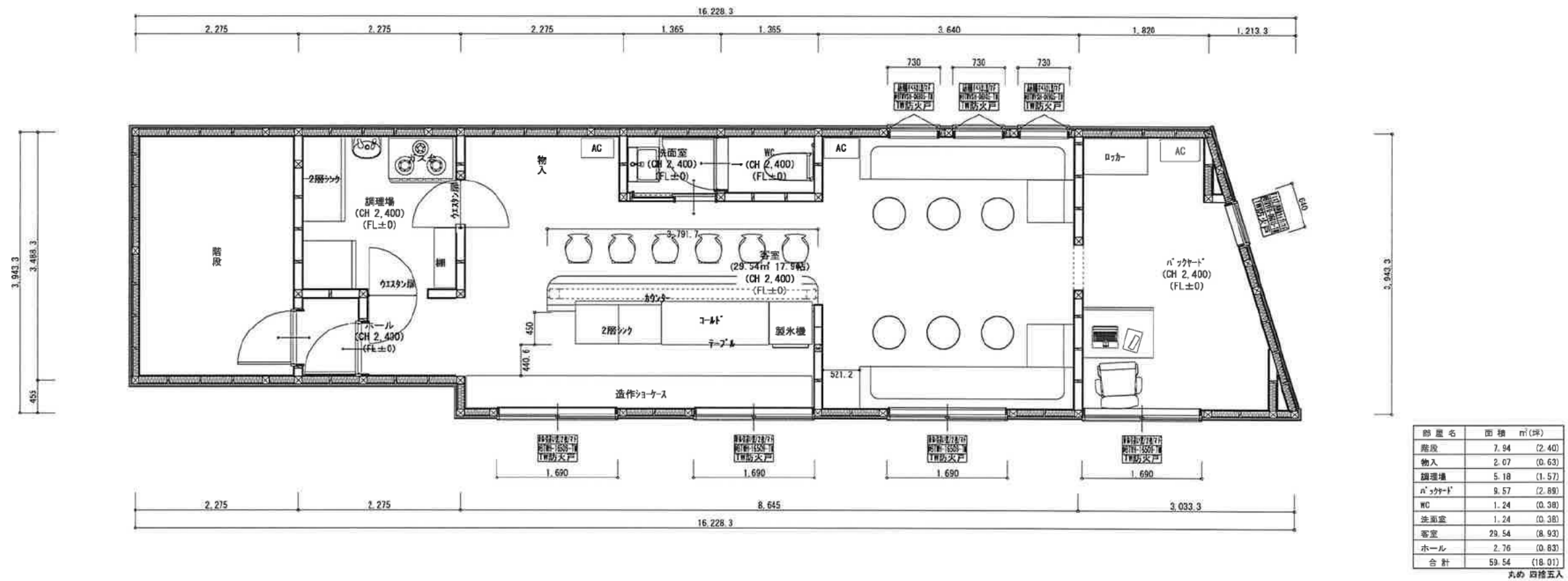
3階 平面詳細図 S:1/70
