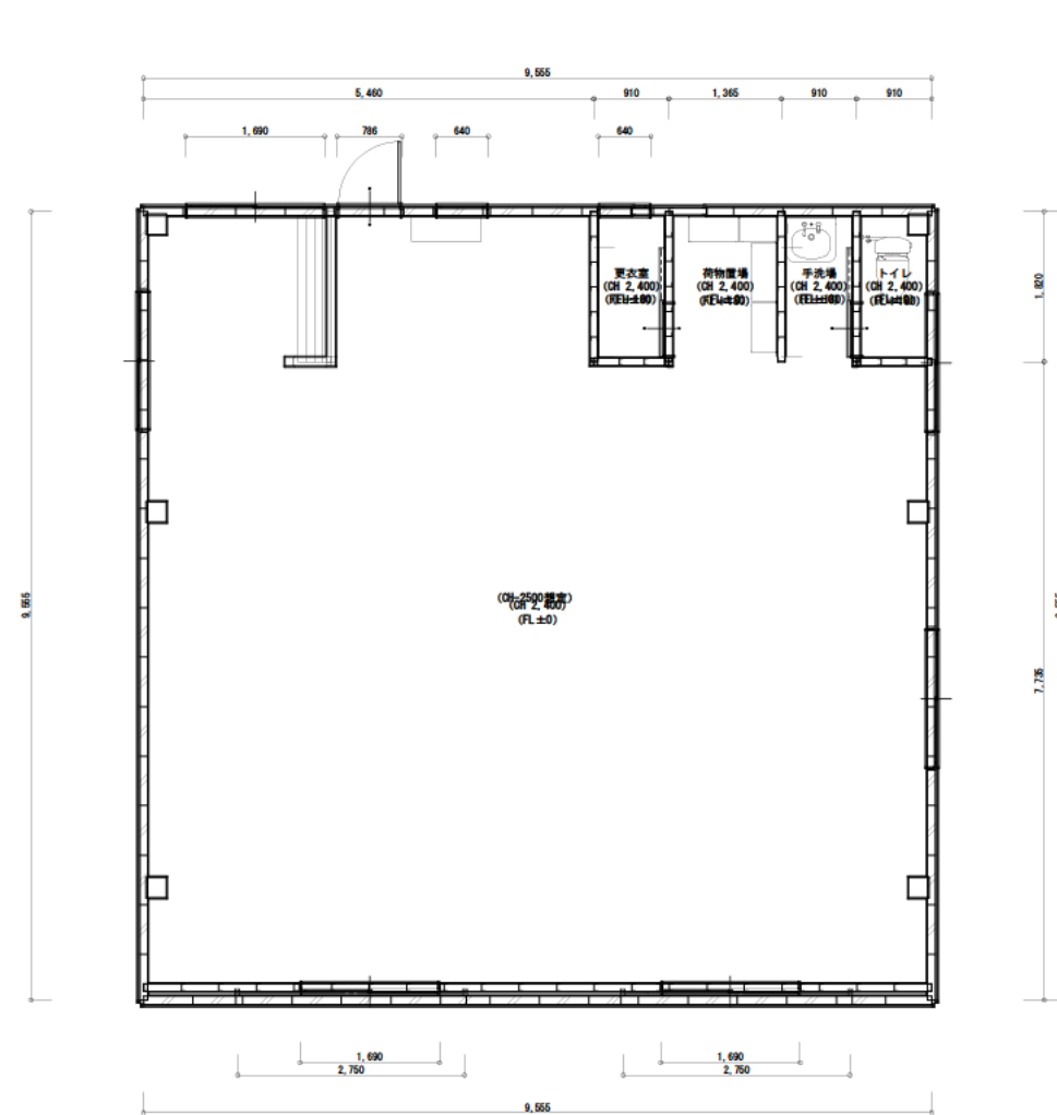
1階 平面詳細図 S:1/100
