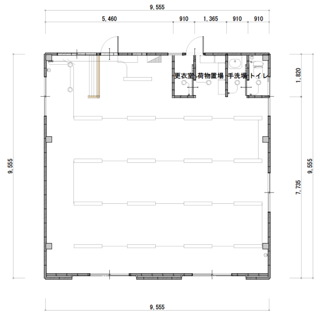
1階 電灯コンセント図 S:1/100
