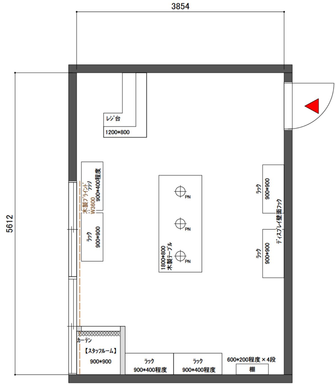
【6F 平面図】
